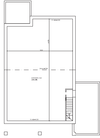
LOTTO 1 - UNITA' 1 PIANTA PIANO SOTTOTETTO Scale 1:100
