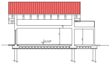
SEZIONE 2-2 scala 1: 100
