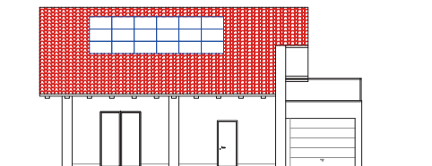
LOTTO 1 - UNITA' 1 PROSPETTO A VALLE NORD-EST Scala 1:100
