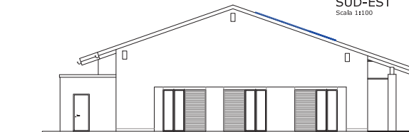
LOTTO 1 - UNITA' 1 PROSPETTO LATERALE SUD-EST Scala 1:100
