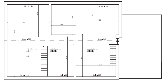
LOTTO 2 - UNITA' 2/1 - 2/2 PIANTA SOTTOTETTO Scala 1:100
