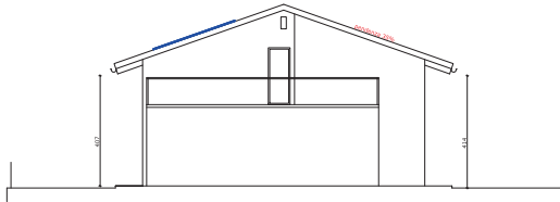
LOTTO 2 - UNITA' 2-1 E 2-2 PROSPETTO A VALLE NORD-EST
