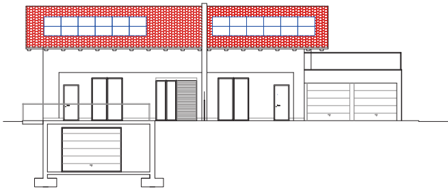
LOTTO 2 - UNITA' 2-1 E 2-2 PROSPETTO A VALLE NORD-EST
