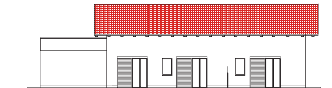
LOTTO 2 - UNITA' 2-1 E 2-2 PROSPETTO A MONTE SUD-OVEST
