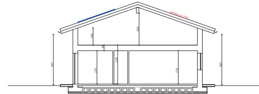
LOTTO 2 - UNITA' 2-1 E 2-2 SEZIONE 2-2
