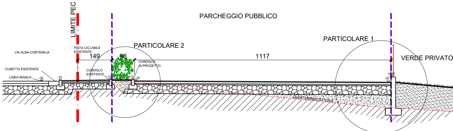
SEZIONE A-A
