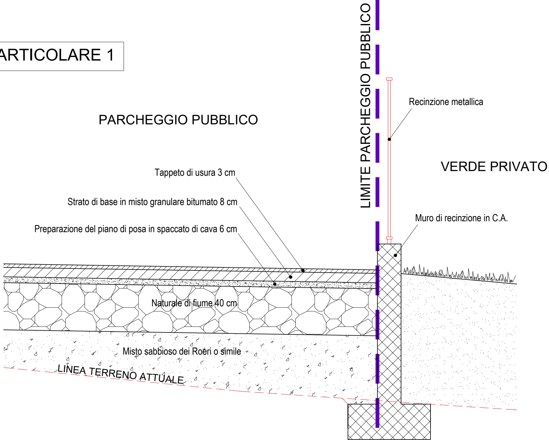
PARTICOLARE 2
