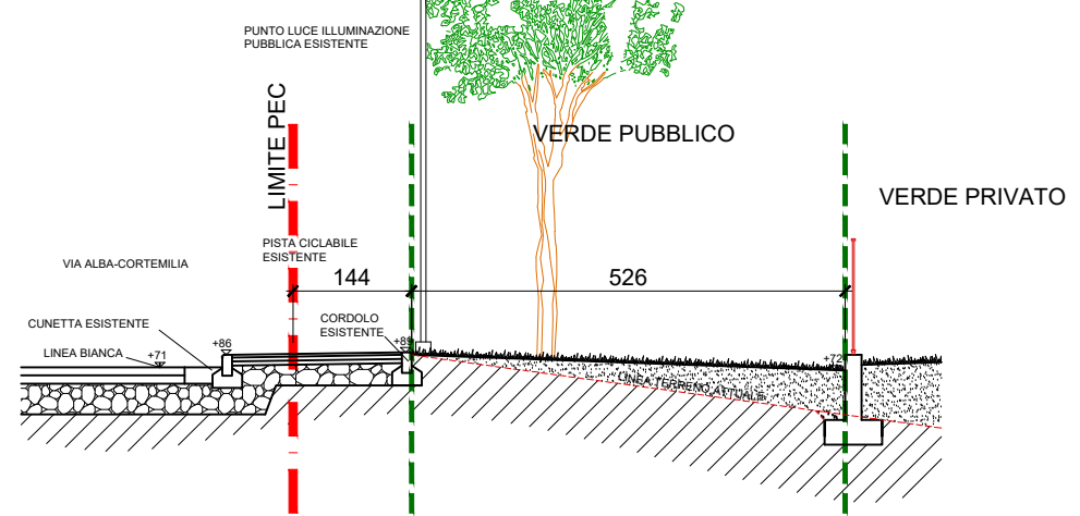
SEZIONE D-D
