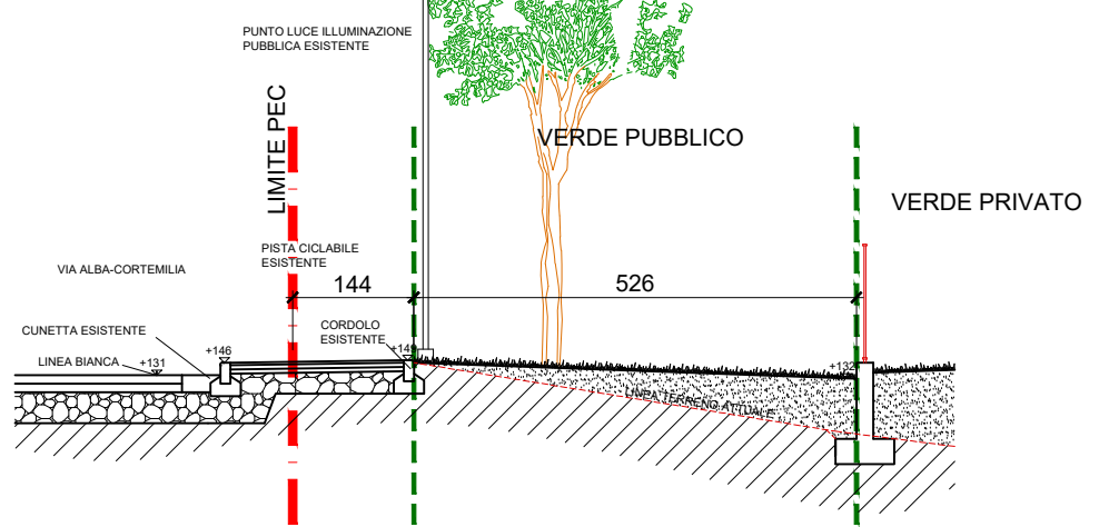
SEZIONE E-E
