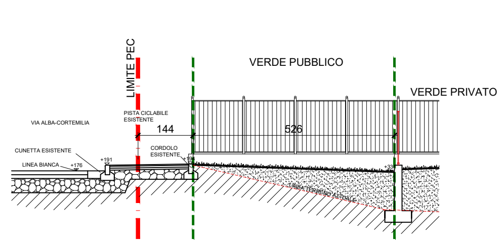
SEZIONE F-F
